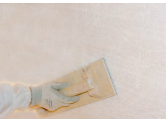
Poncer la surface de la façade EPS
