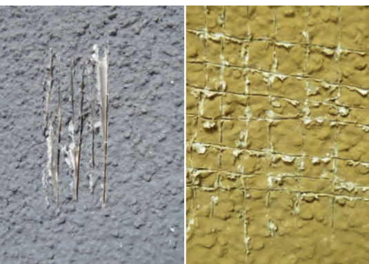
Photo gauche : coupe parallèle/couche insuffisamment porteuse
