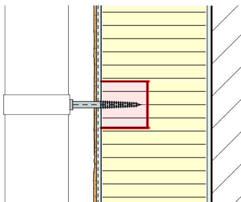
63 Cylindre de montage ZyRillo® Ø 70 mm
