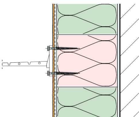
64 Carreau de montage Quadroline® EPS 150 x 100 mm (collé sur le support avec la colle du système)
